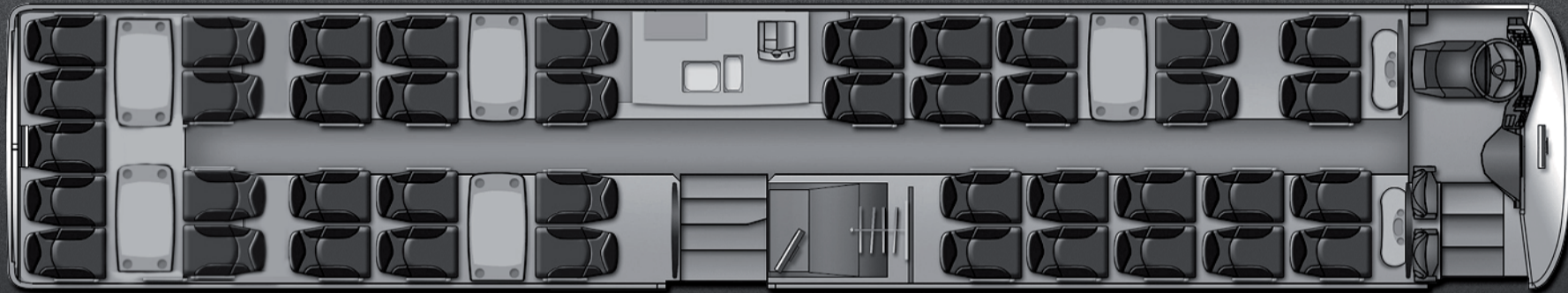
Floorplan Mercedes-Benz Travego S41/1 (41 Sitzplätze - davon 20 Plätze an Tischen)
